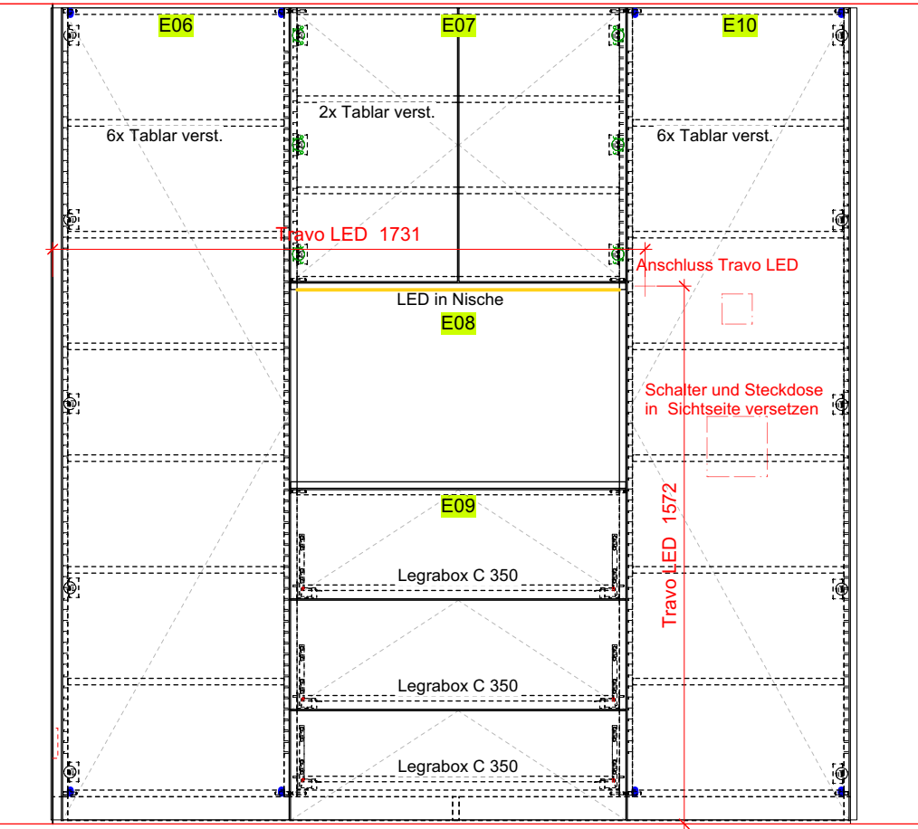
Ansicht Wohnen
