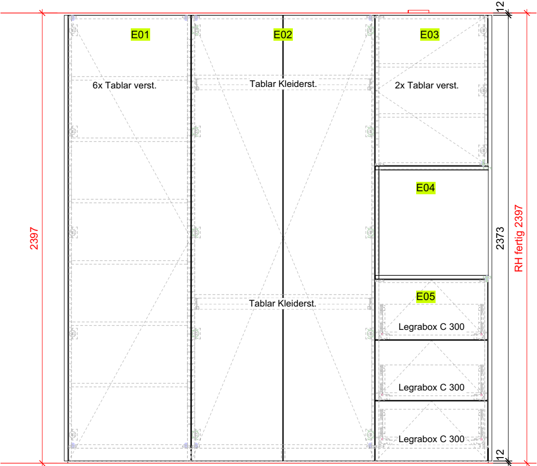
Ansicht Korridor
